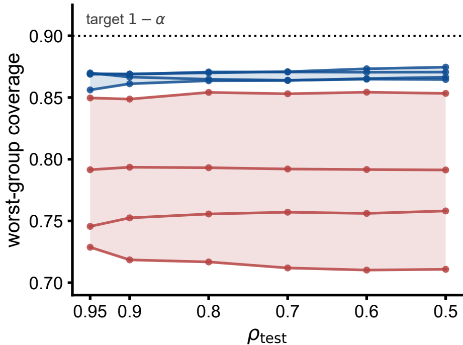
Waterbirds
