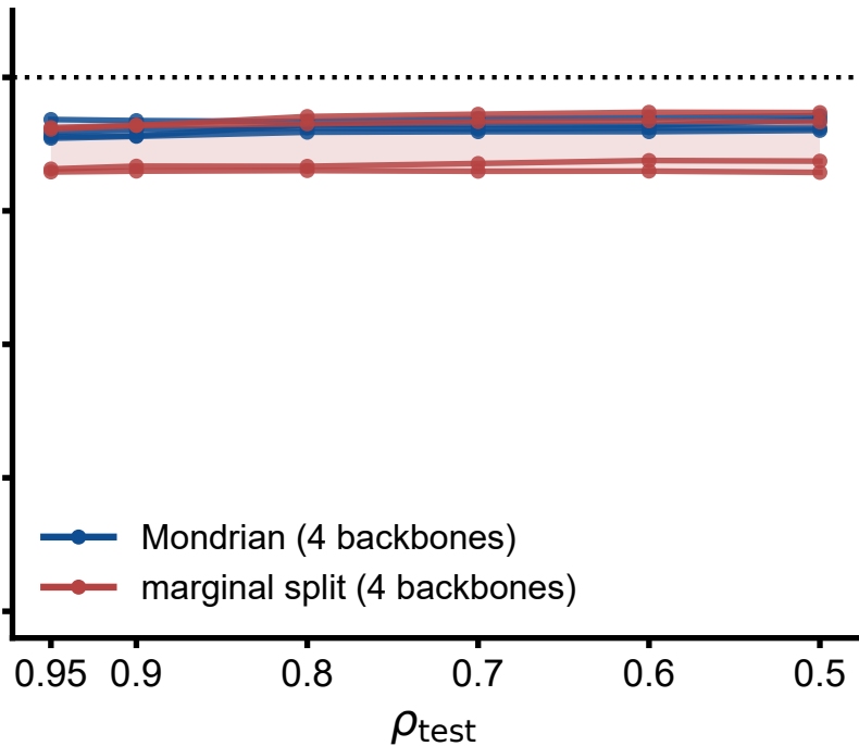
CelebA
